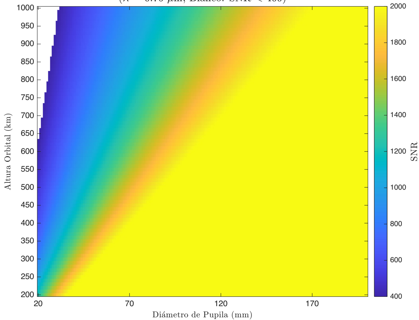
SNR - Refractivo - Detector 1 ( \lambda = 0.76 \mu\text{m} , Blanco: SNR < 400)
